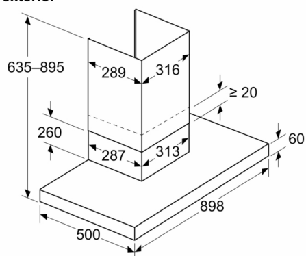
Dimensiones en mm Aparato en modo de salida de aire al exterior
