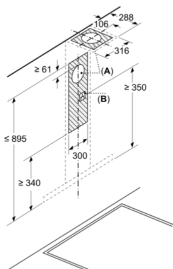
Dimensiones en mm
