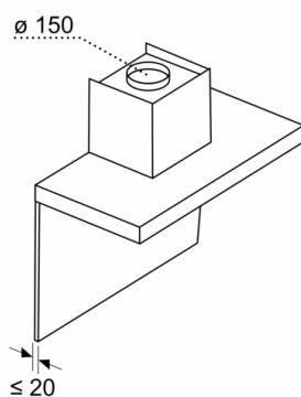
Dimensiones en mm Profundidad del panel
