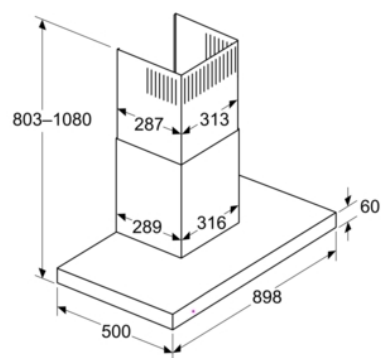
Dimensiones en mm Perspectiva de recirculación
